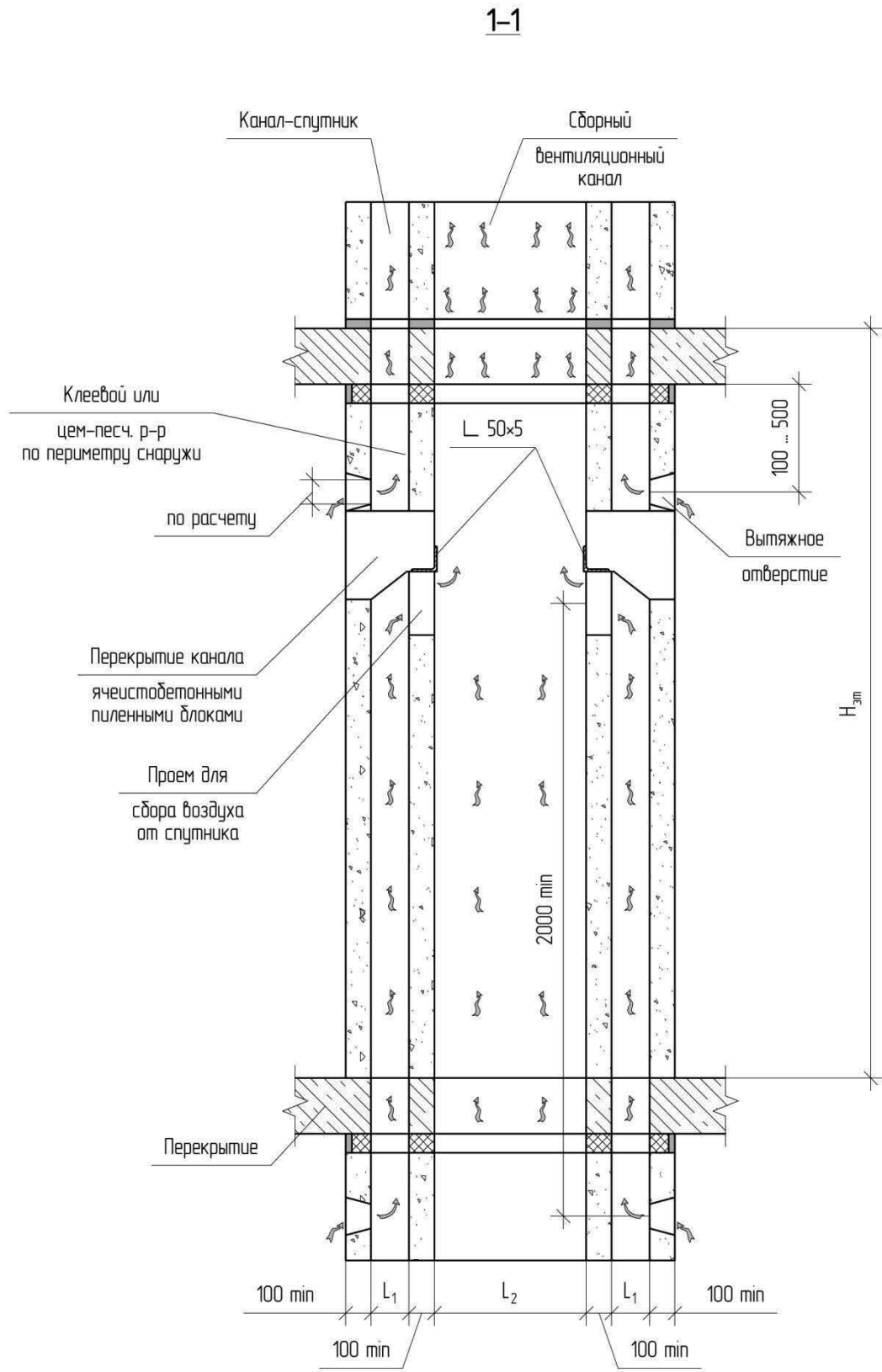
Узел XIII. Устройство вентиляционных шахт
