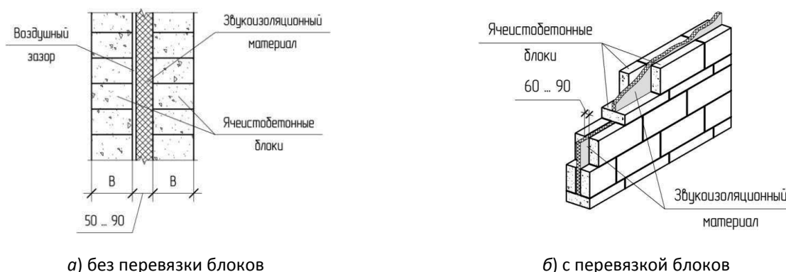
Рис. 3.5. Примеры устройства стен со звукоизоляционной прослойкой
