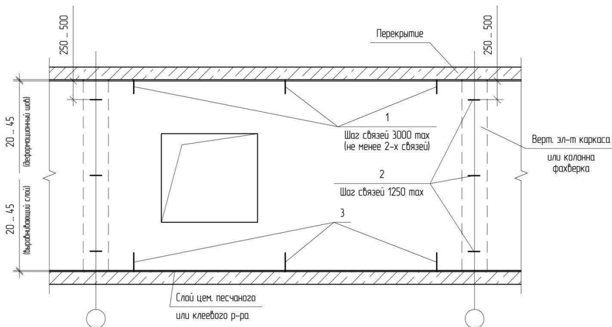
Рис. 4.5. Схема расположения связей (креплений) наружных и внутренних стен
