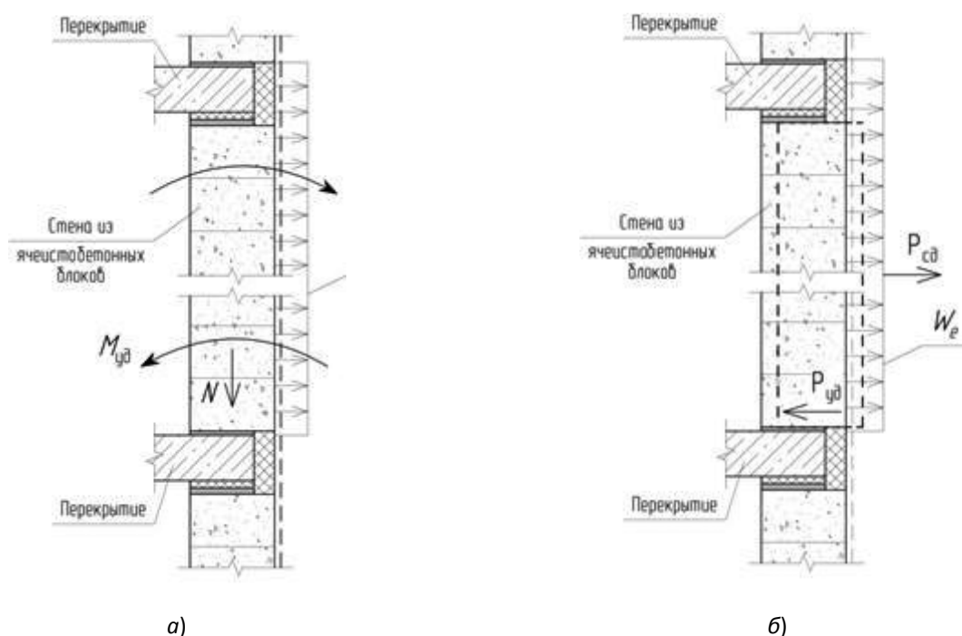
Рис. 3.13. Расчетные схемы поэтажно опертой стены
