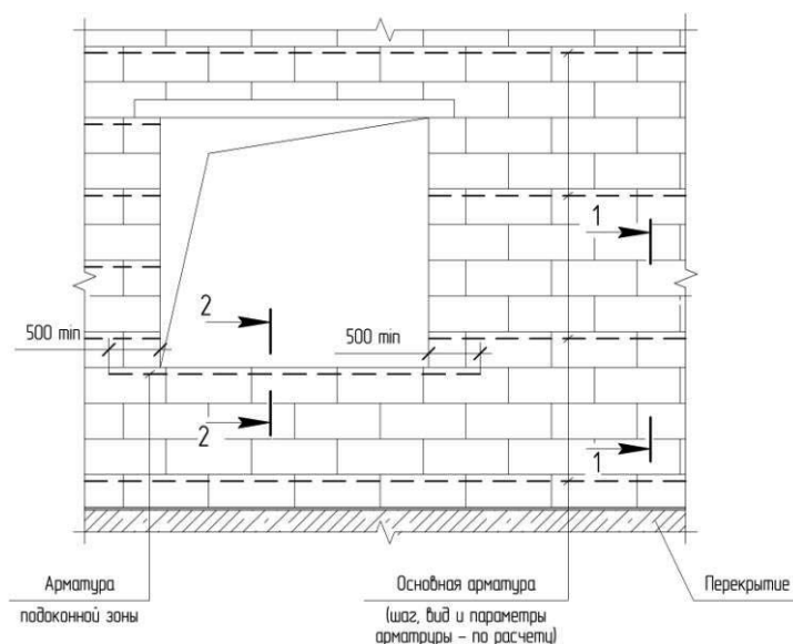
Рис. 3.6. Пример схемы армирования стен
