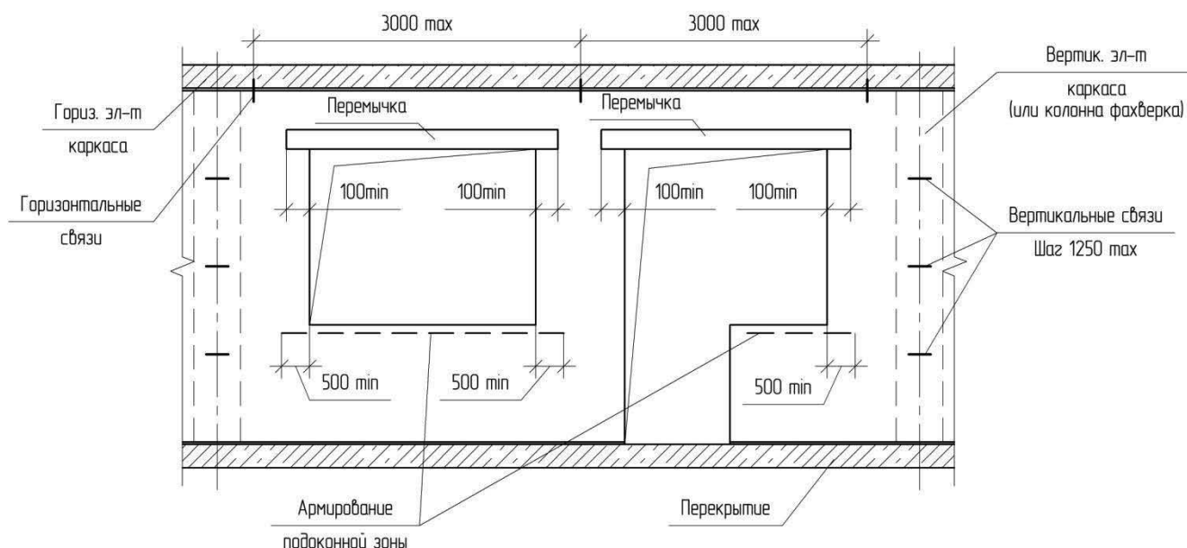
Рис. 4.8. Схема устройства проемов на примере наружной стены
