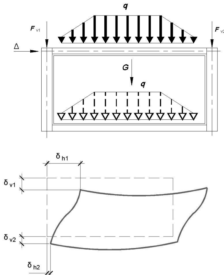
Рис. 3.12. Схемы для определения нагрузок
